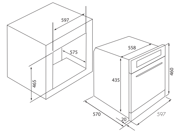
BAO4636-P : 15 AMP PLUG
