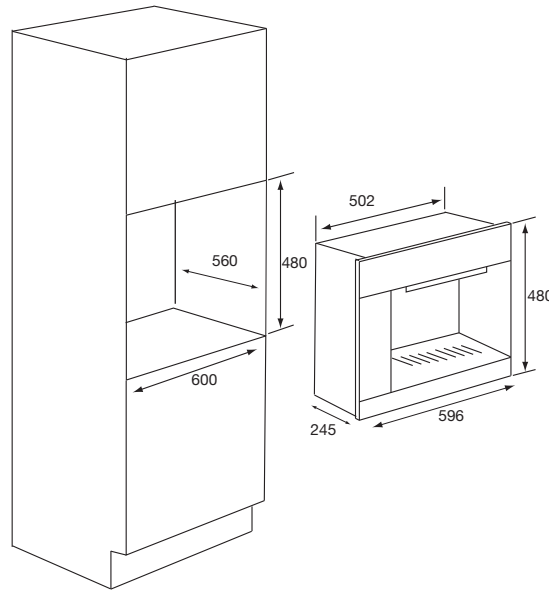
BAEC2SS : 10 AMP PLUG
