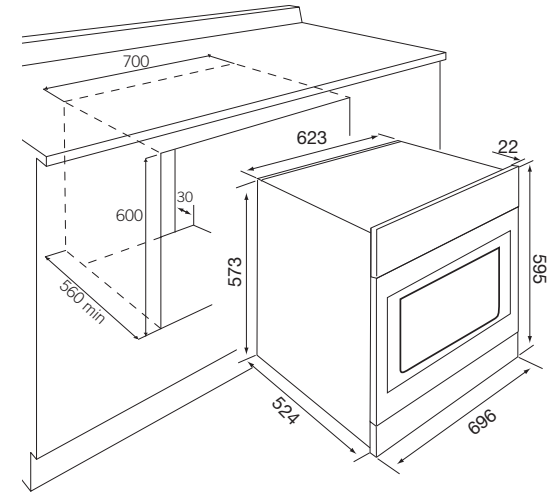
BAO7006-P : 15 AMP PLUG
